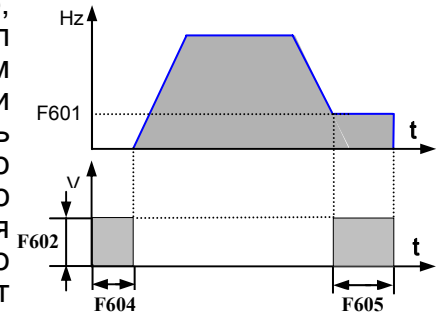
Рис 5-9 Торможение
